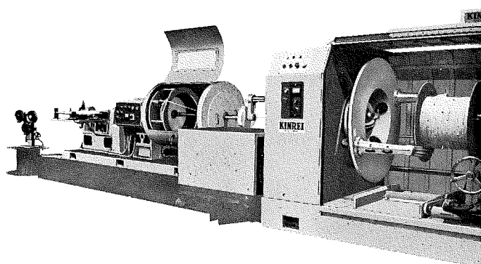
縦添テープ+センター巻テープシステム
