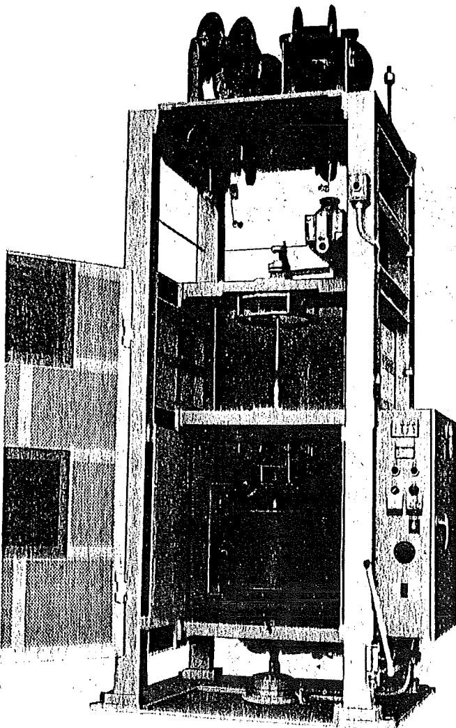
φ300 × 4 B 4ヶ撚機
